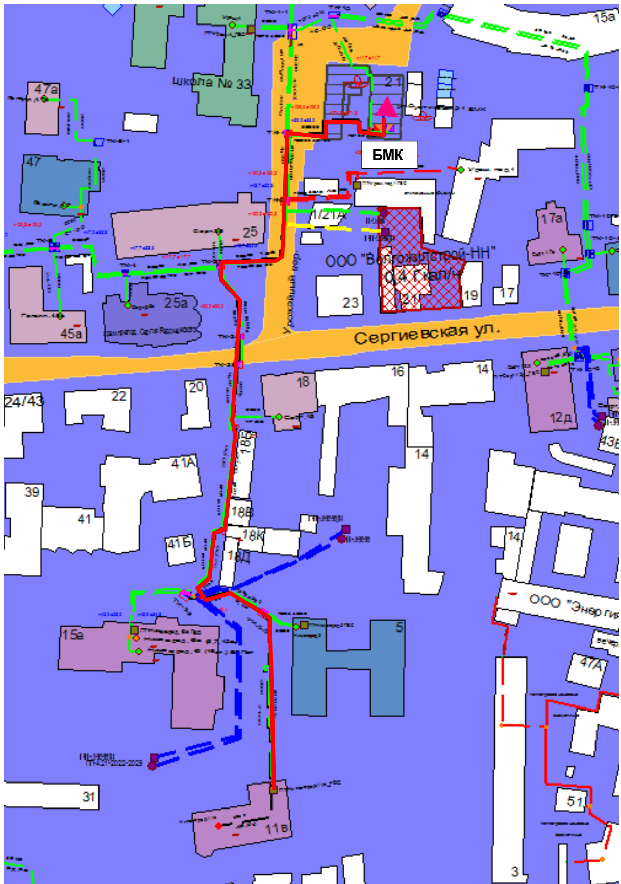
Рисунок 0.9 – Результат гидравлического расчета - расчетный путь теплоносителя от котельной Суетинская, 21 до ПТ-НТжгород, 11в
