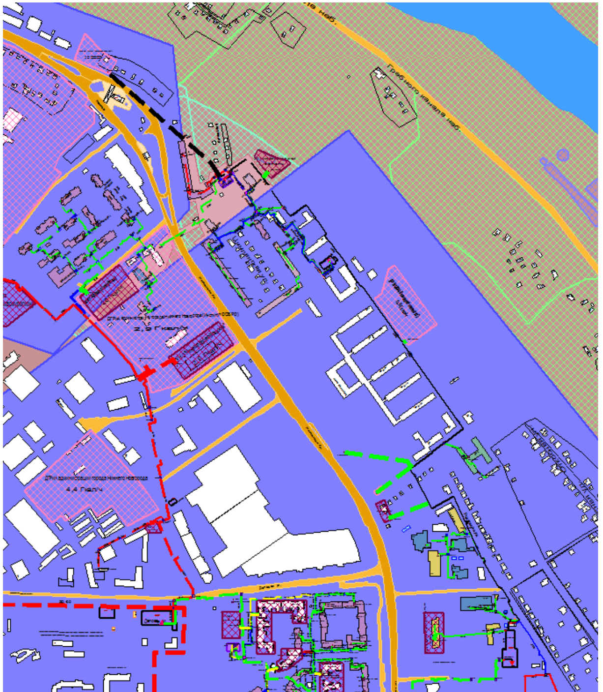
Рисунок 0.71 – Результат гидравлического расчета - расчетный путь теплоносителя от котельной ул. Родионова, 1946 до ПТ-ПП-2.67-2017
