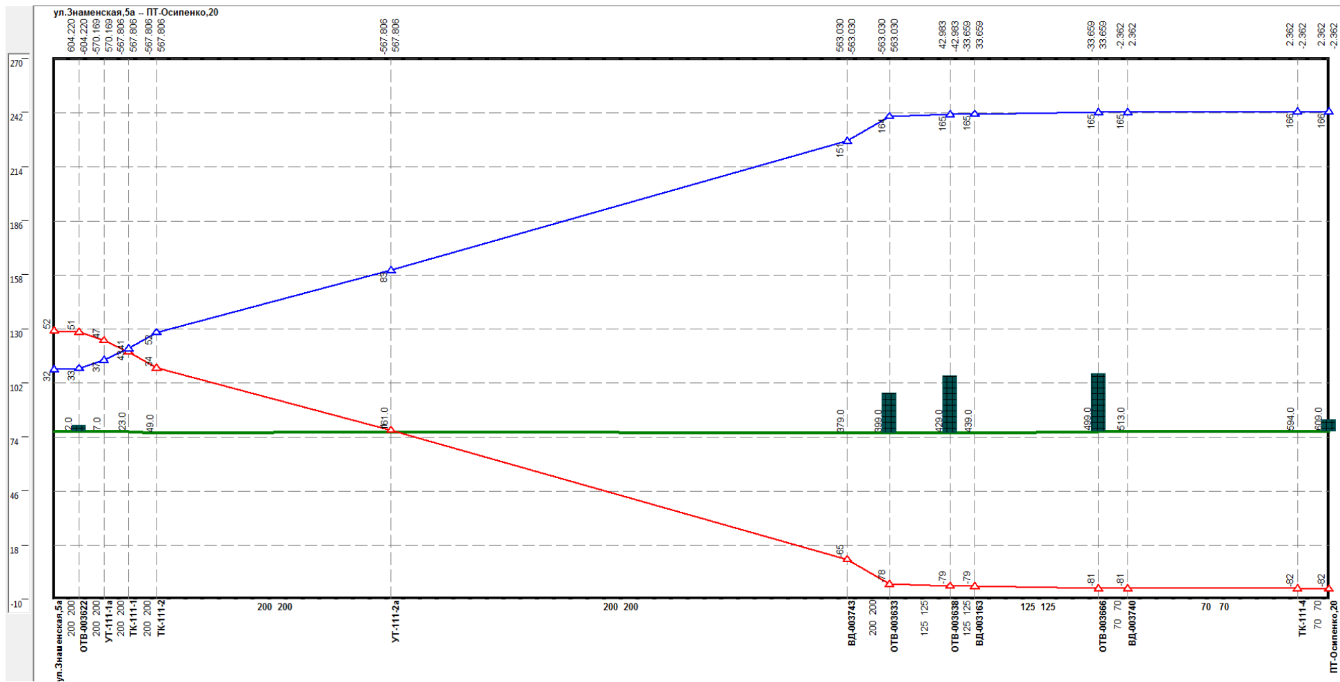
Рисунок 0.22 –Результат гидравлического расчета - график гидравлических режимов по пути теплоносителя от Знаменская 5а до ПТ-Осипенко,20
