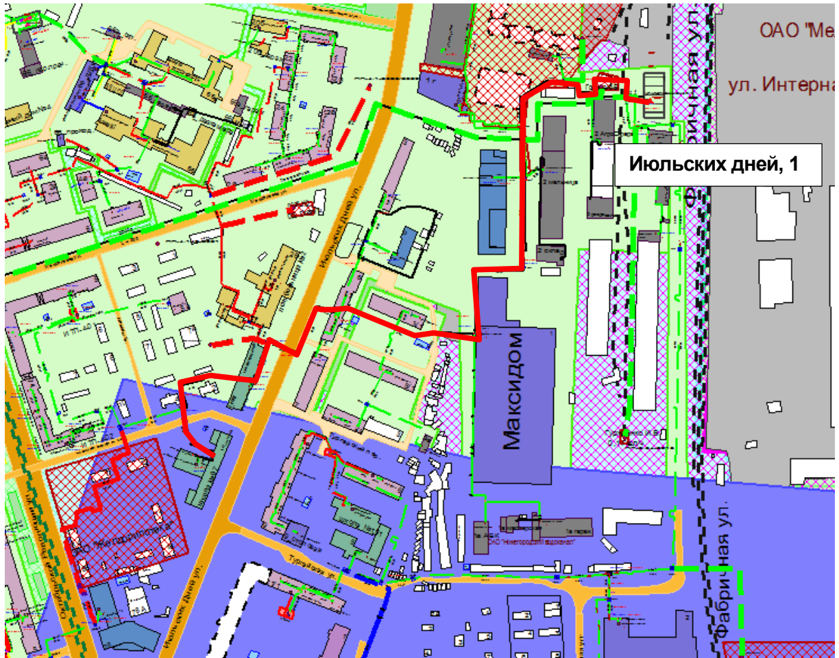
Рисунок 0.31 – Результат гидравлического расчета - расчетный путь теплоносителя от Июльских дней, 1 до ПТ-Июль.дней, 10 школа
