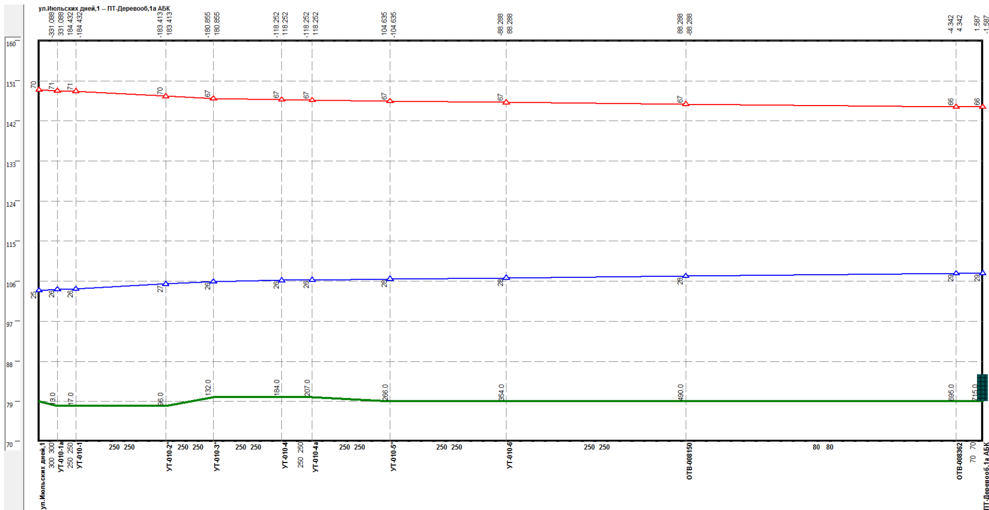
Рисунок 0.97 –Результат гидравлического расчета - график гидравлических режимов по пути теплоносителя от котельной Июльских дней, 1 до ПТ-Деревооб,1а АБК
