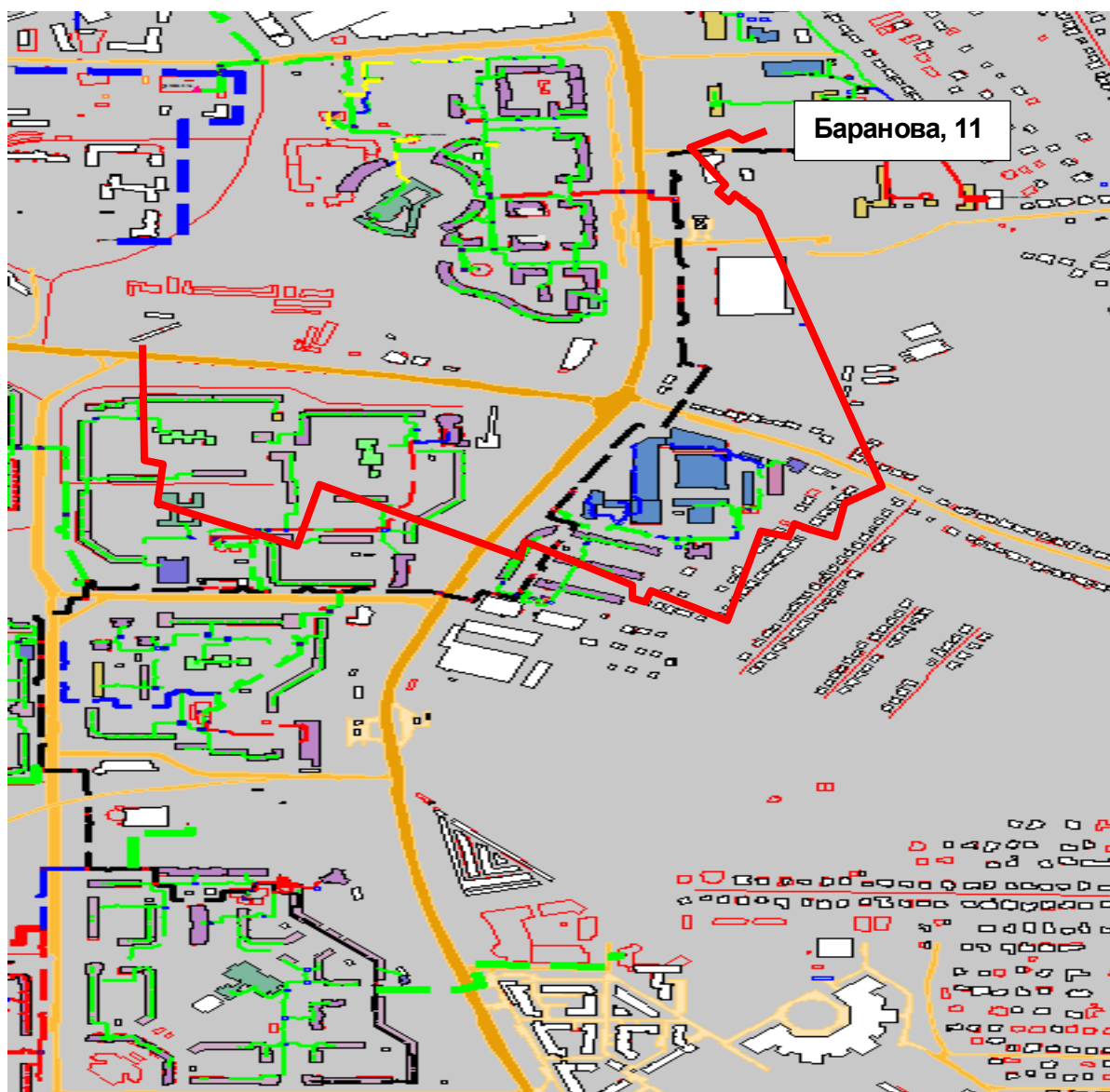
Рисунок 0.100 – Результат гидравлического расчета - расчетный путь теплоносителя от котельной ул. Родионова, 1946 до ПТ-Богдан.1 пр.
