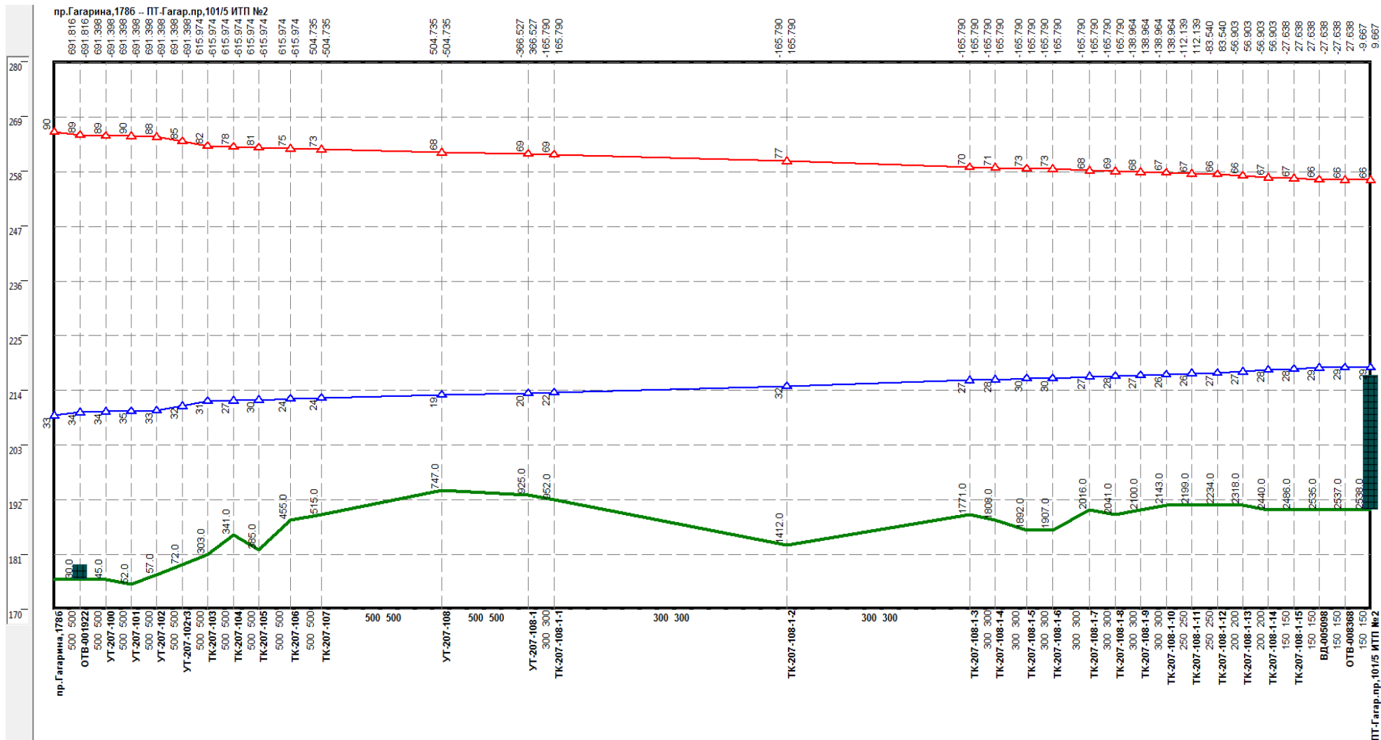
Рисунок 0.70 –Результат гидравлического расчета - график гидравлических режимов по пути теплоносителя от котельной пр. Гагарина, 1786 до ПТ-Гагар.пр.101/5 ИТП №2.
