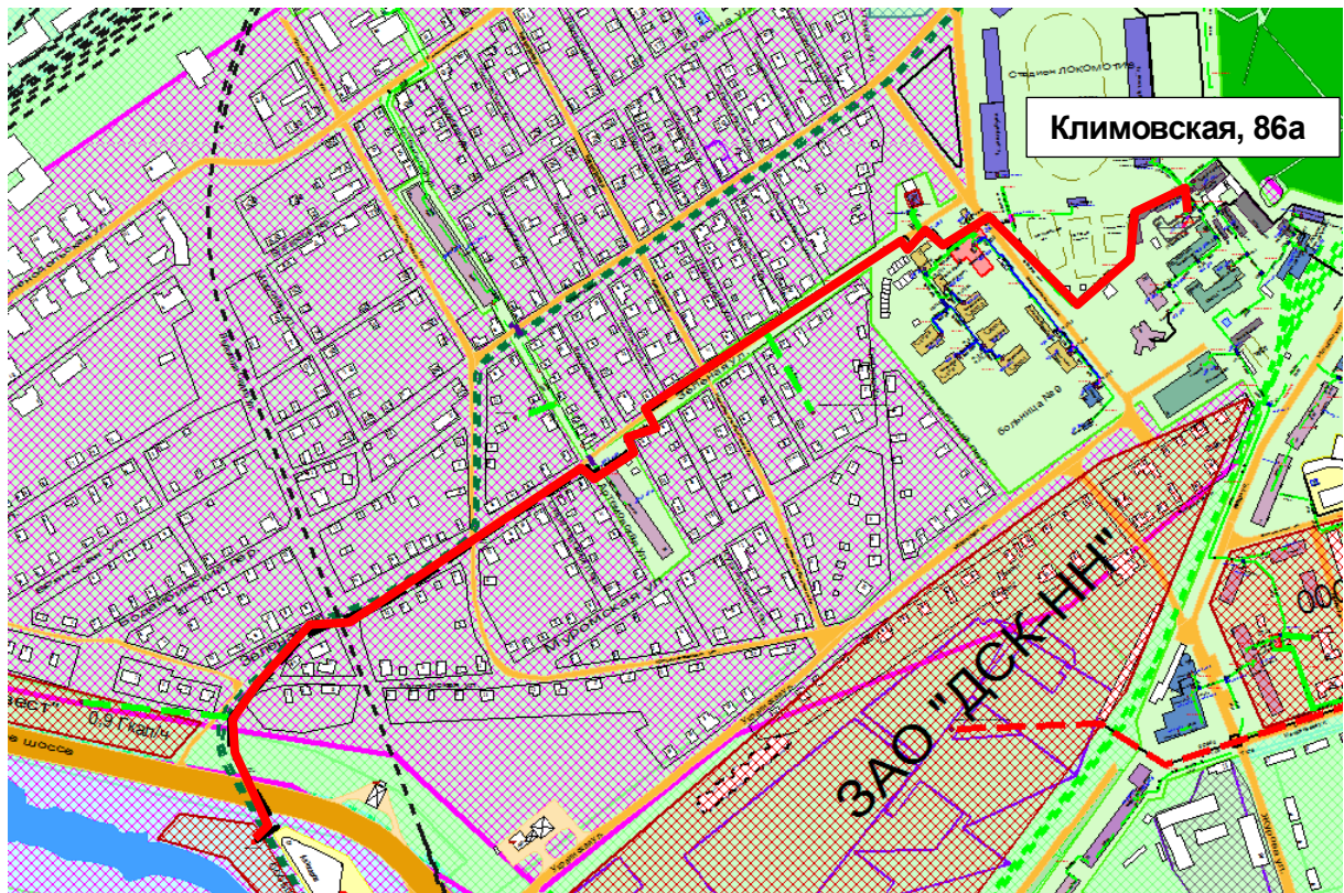
Рисунок 0.45 – Результат гидравлического расчета - расчетный путь теплоносителя от котельной Климовская, 86а до ПТ-ПП-2.227-2016
