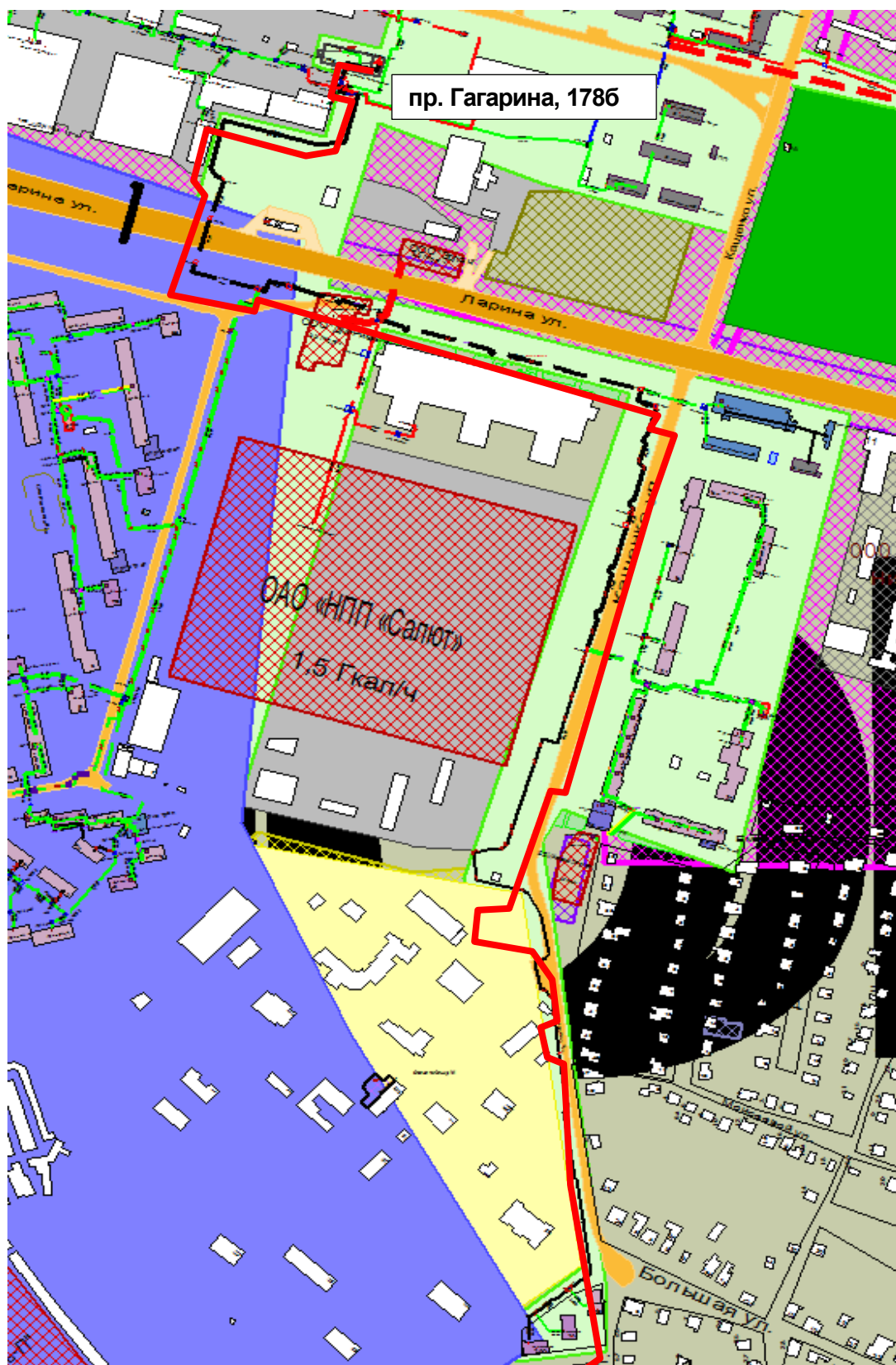
Рисунок 0.112 – Результат гидравлического расчета - расчетный путь теплоносителя от котельной пр. Гагарина, 1786 до ПТ-Кашенко, 4а
