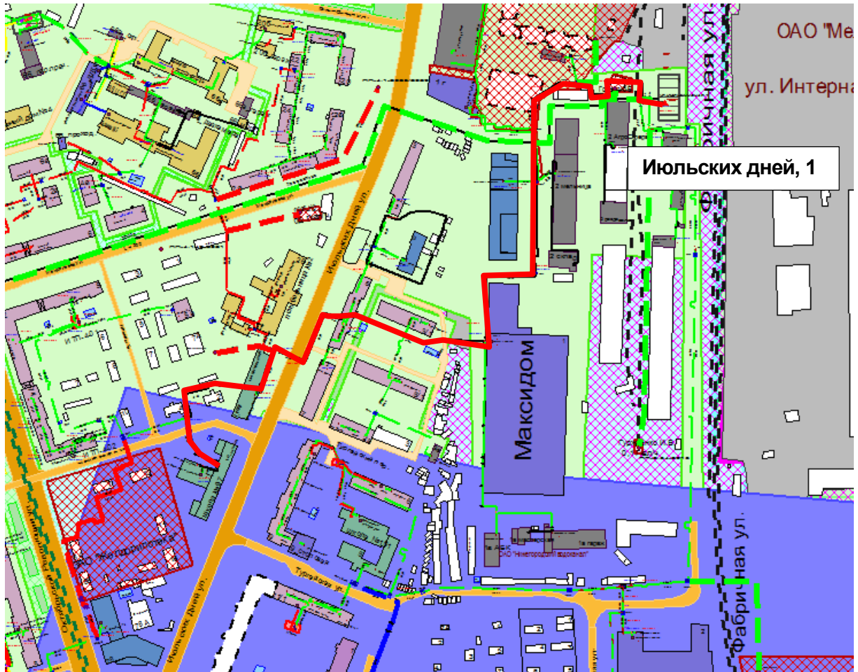
Рисунок 0.94 – Результат гидравлического расчета - расчетный путь теплоносителя от Июльских дней, 1 до ПТ-Июль.дней, 10 школа
