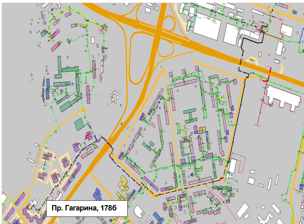
Рисунок 0.69 – Результат гидравлического расчета - расчетный путь теплоносителя от котельной пр. Гагарина, 1786 до ПТ-Гагар.пр.101/5 ИТП №2.
