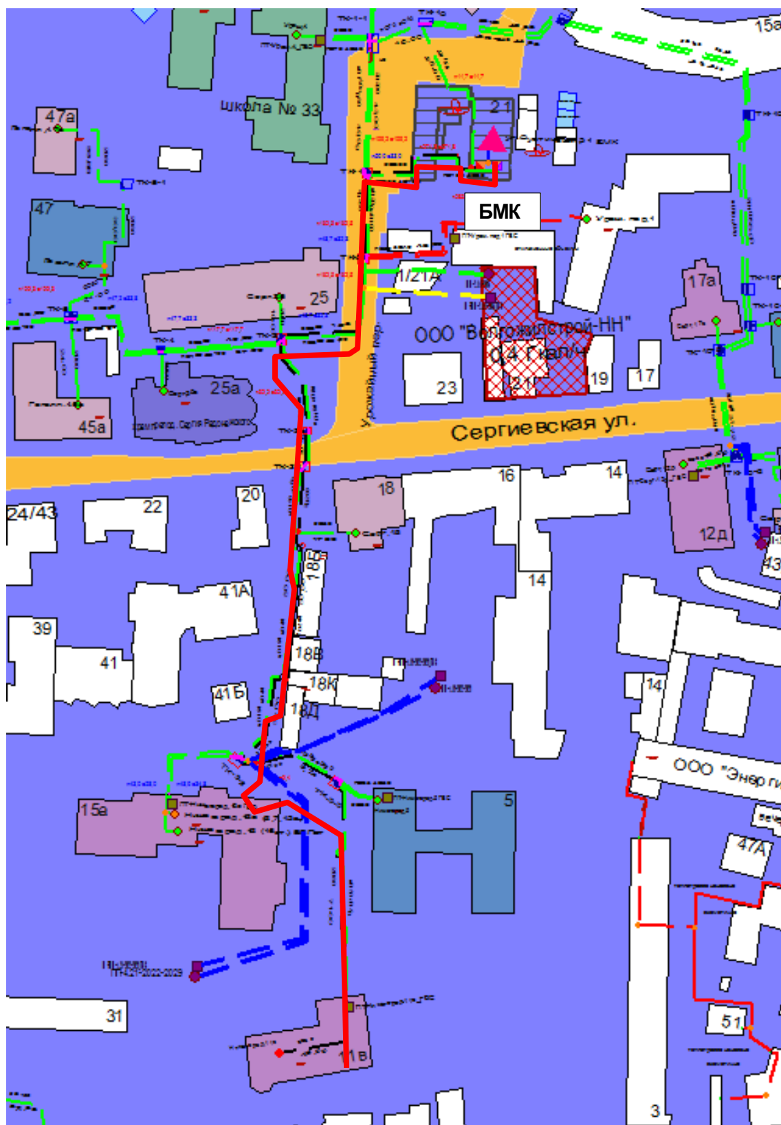
Рисунок 0.82 – Результат гидравлического расчета - расчетный путь теплоносителя от котельной Суевинская, 21 до ПТ-Нтжегород, 11в
